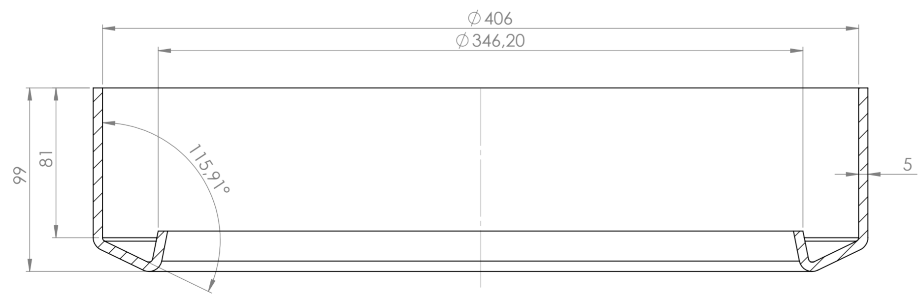
ŘEZ A-A MĚŘITKO 1 : 2
